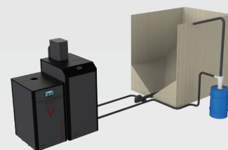
Vakuumtransport mit Pelletlager aus Eigenbau
